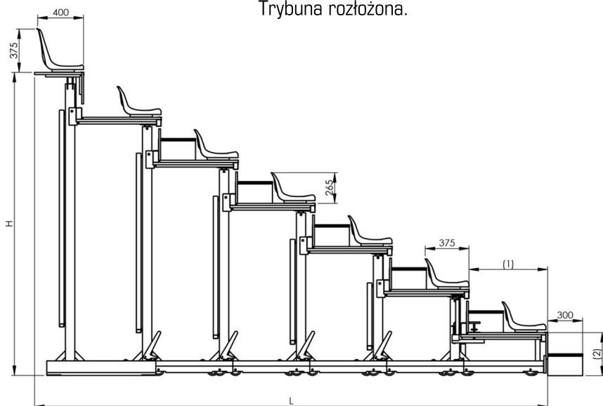
Trybuna rozłożona.
